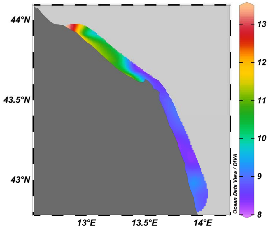
Ossigeno disciolto (mg/L) sul fondo
